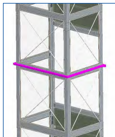
FISSAGGIO AD ANELLO RING FIXING
